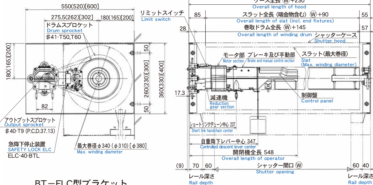
BT-ELC型ブラケット Bracket Type BT-ELC
