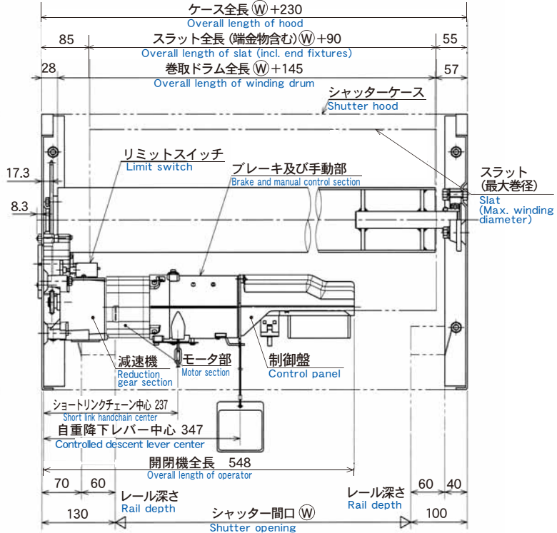
BC-ELC型ブラケット Bracket Type BC-ELC
