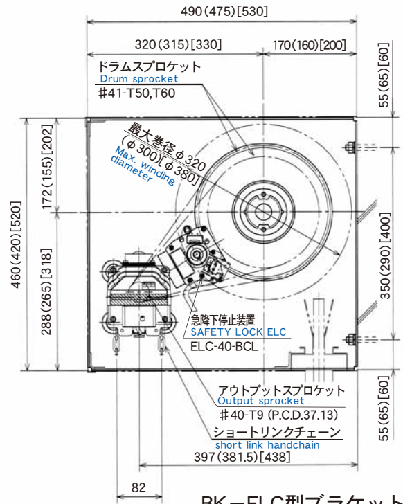
BK-ELC型ブラケット Bracket Type BK-ELC
