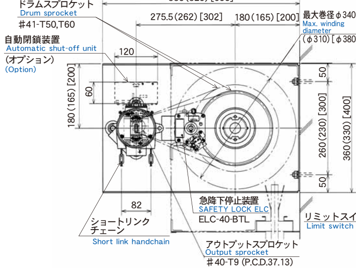
BT-ELC型ブラケット Bracket Type BT-ELC
