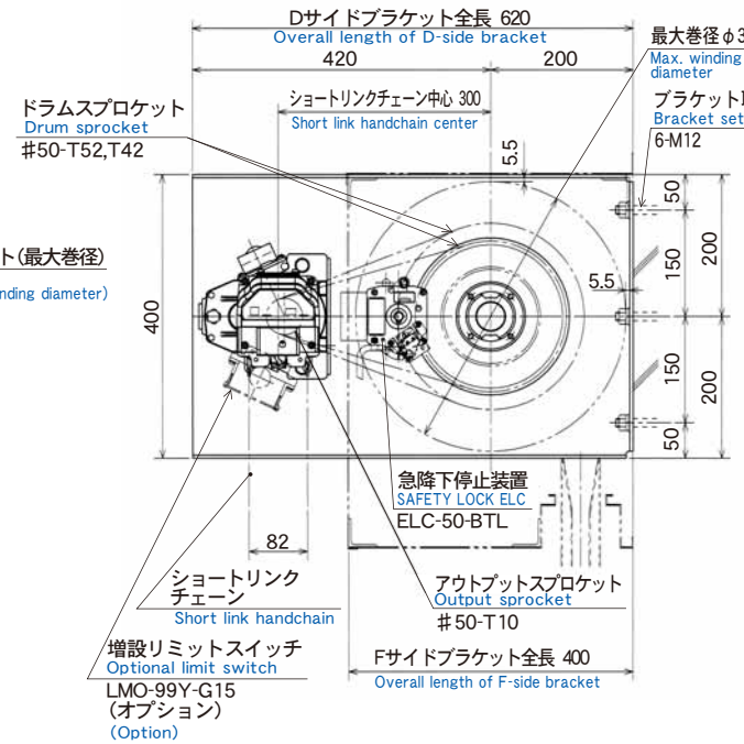
BT-25M-ELC型ブラケット Bracket Type BT-25M-ELC
